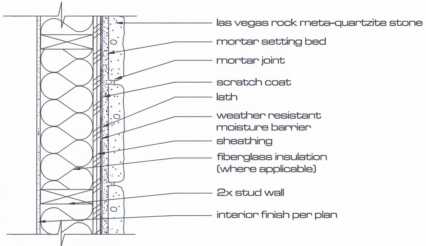
○ meta-quartzite stone over sheathing over studs scale: n.t.s.
